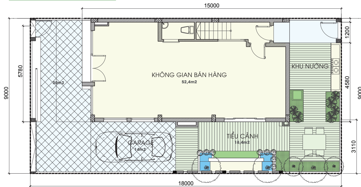
Mặt bằng Tầng 1 mẫu P1-1
