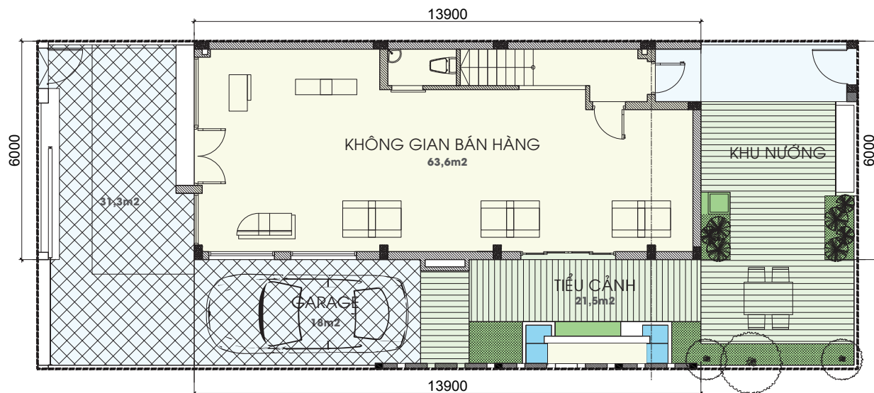
Mặt bằng Tầng 1 mẫu P1-3
