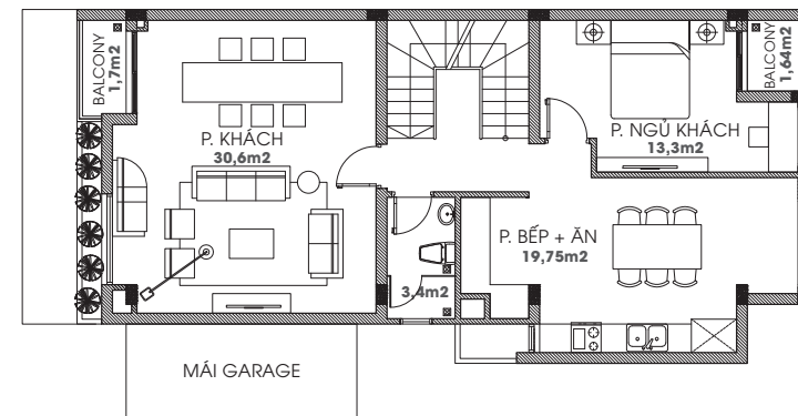
Mặt bằng Tầng 3
