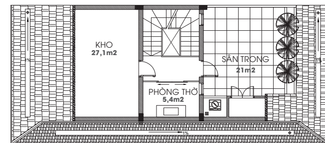
Mặt bằng Tầng áp mái
