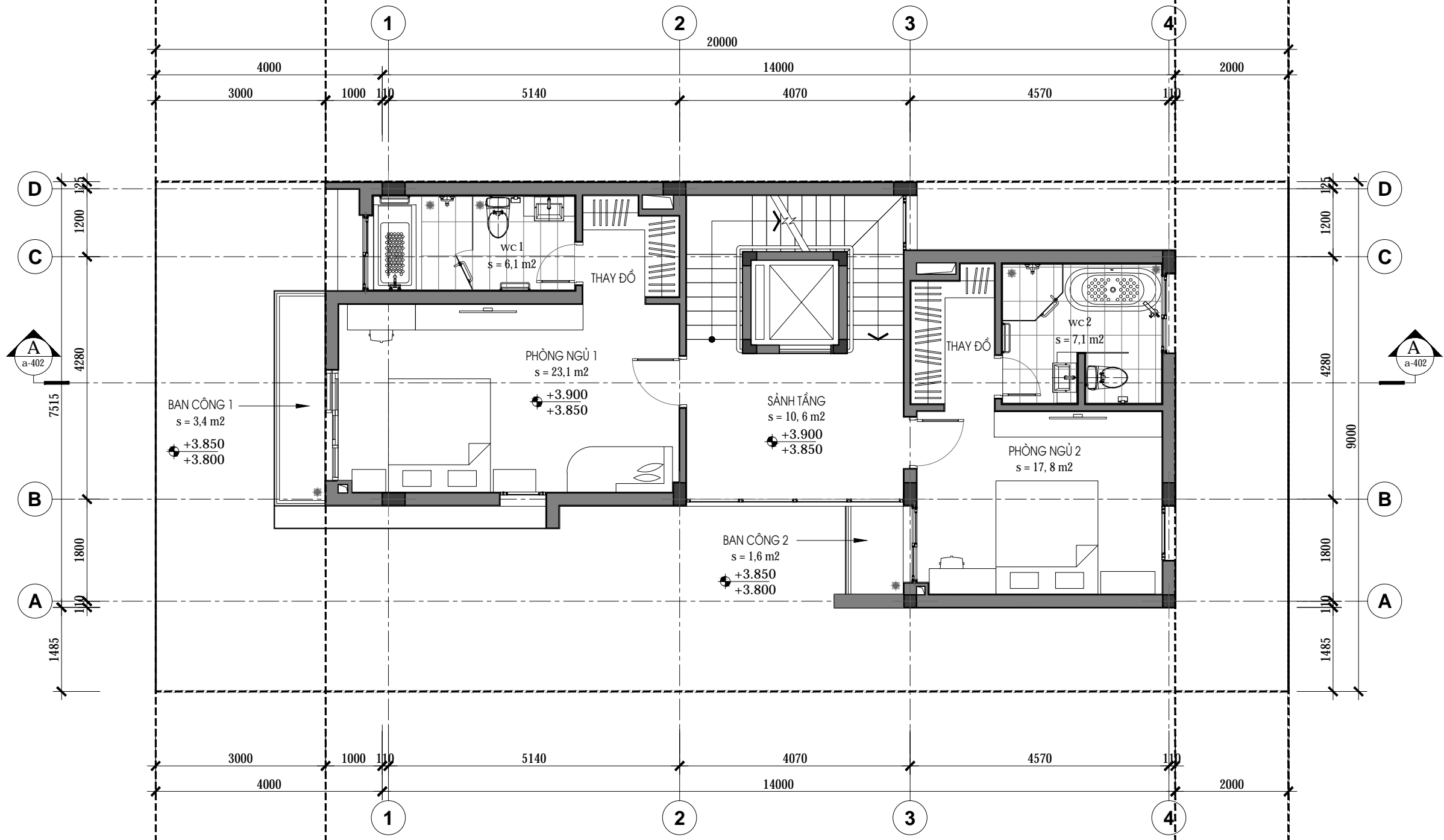
MẶT BẰNG TẦNG 2 TỶ LỆ: 1/75
