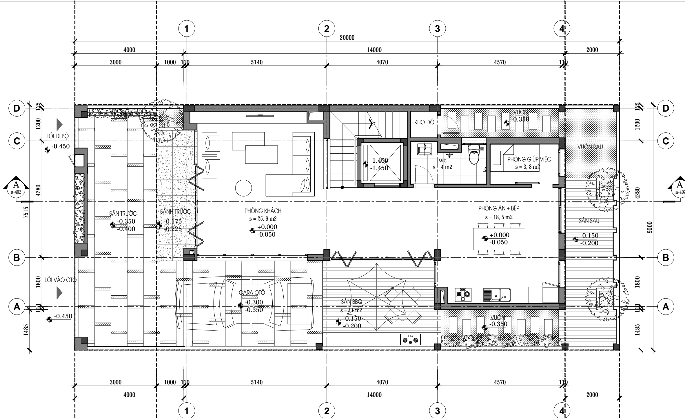
MẶT BẰNG TẦNG 1 TỶ LỆ: 1/75
