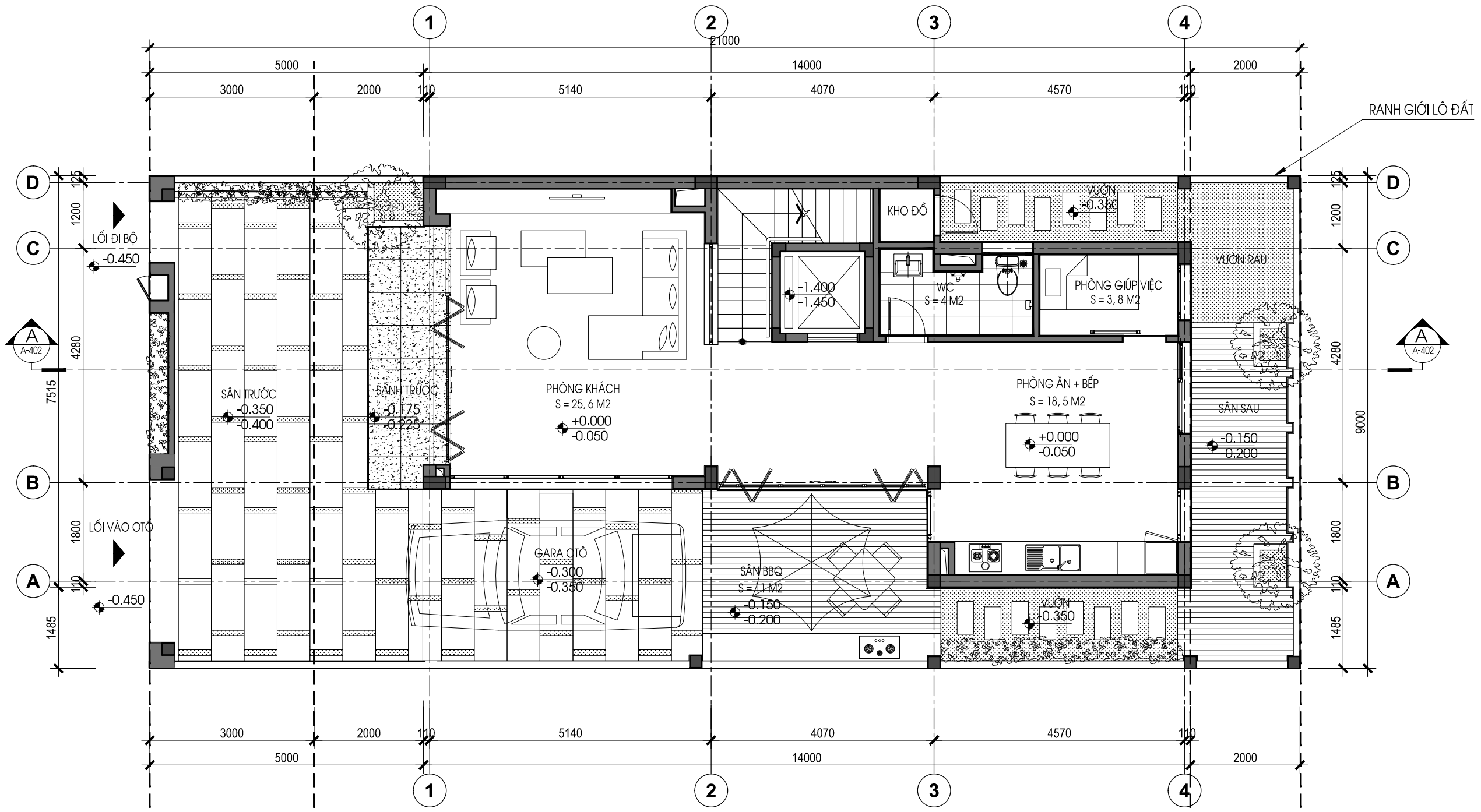
MẶT BẰNG TẦNG 1 TỶ LỆ: 1/75
